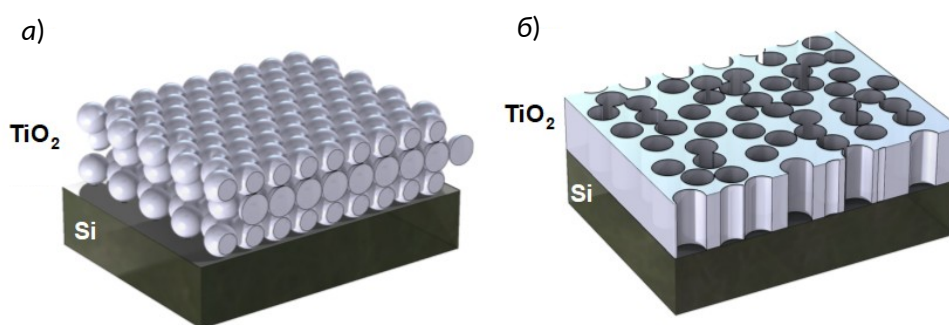
Рисунок 1 - Структурные типы АО-слоя для моделирования оптического пропускания СЭ: самосборка \text{TiO}_2 наносфер (а) и случайное распределение вертикальных нанопор (б)
