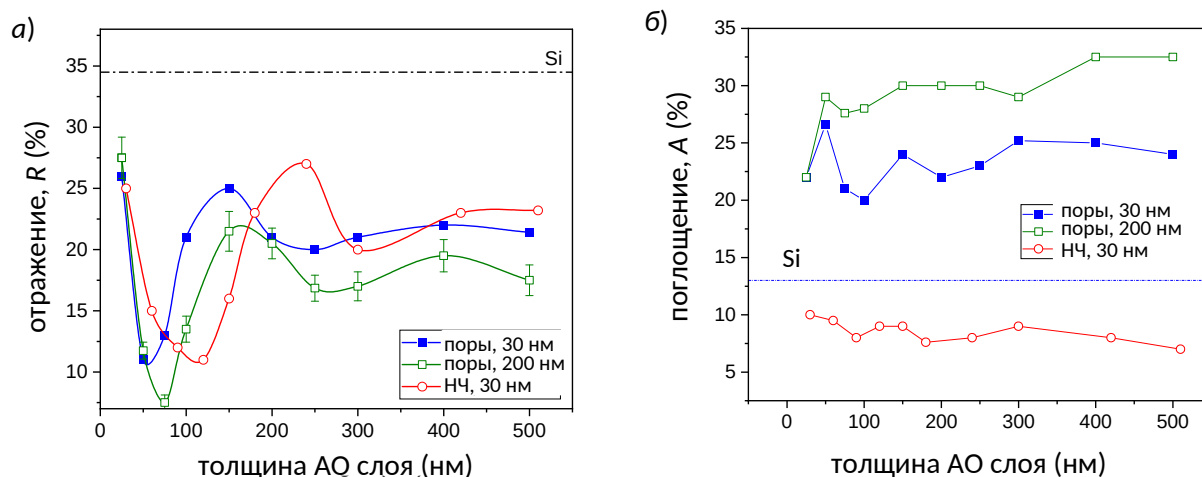
Рисунок 3 - Зависимость коэффициентов отражения R(\lambda) и поглощения A(\lambda) от толщины АО слоя двух структурных типов
