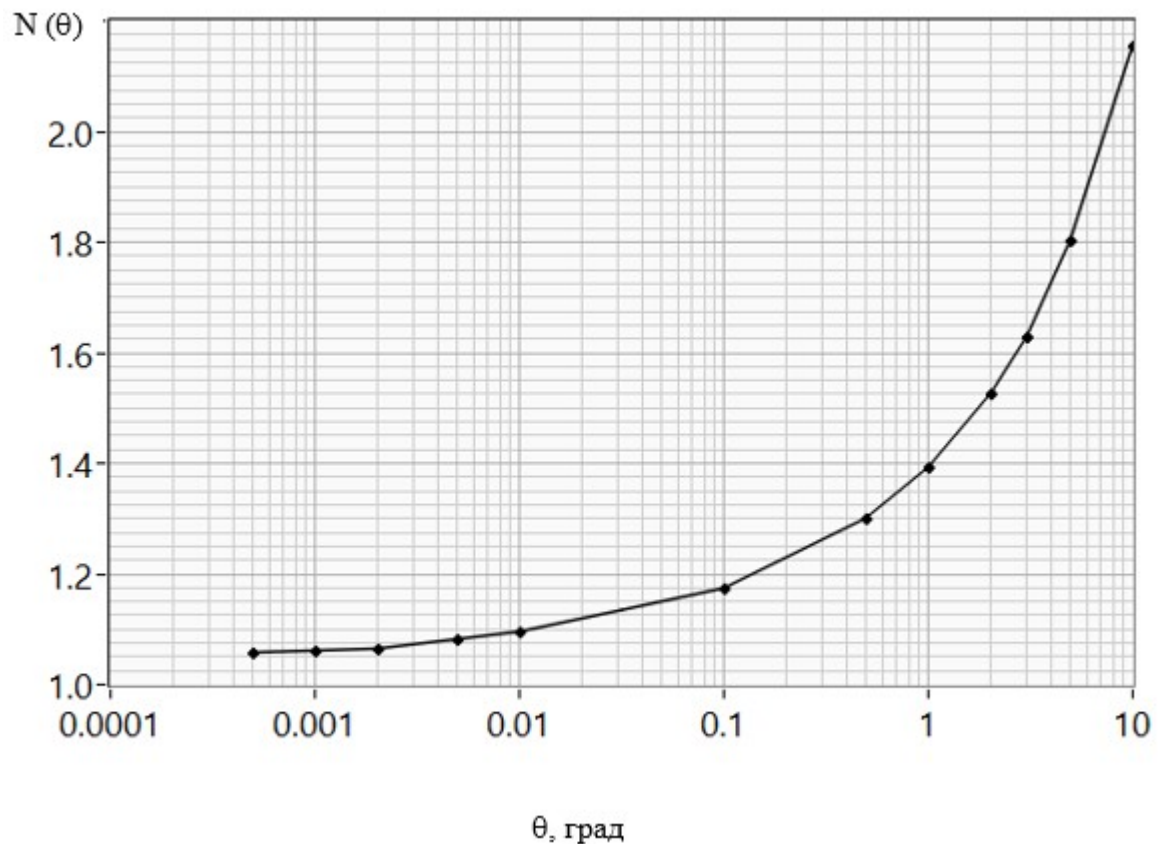
Рисунок 1 – Отношение показателей степени в экспоненциальном сомножителе в (1) и в (3) как функция углового разноса точек наблюдения
