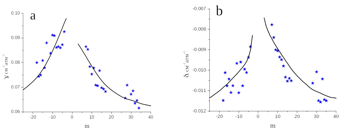
Рисунок 1 – Экспериментальные (звездочки) и вычисленные (линия) коэффициенты уширения (а) и сдвига (б) линий закиси азота давлением воздуха в полосе 3\nu_1+4\nu_3
