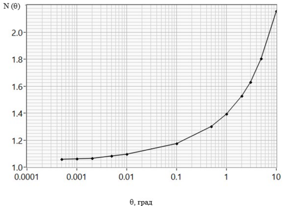
Рисунок 1 – Отношение показателей степени в экспоненциальном множителе в (1) и в (3) как функция углового разноса точек наблюдения
